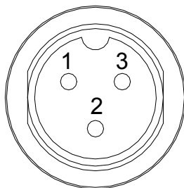
图 4-2 遥控口插座（公）
