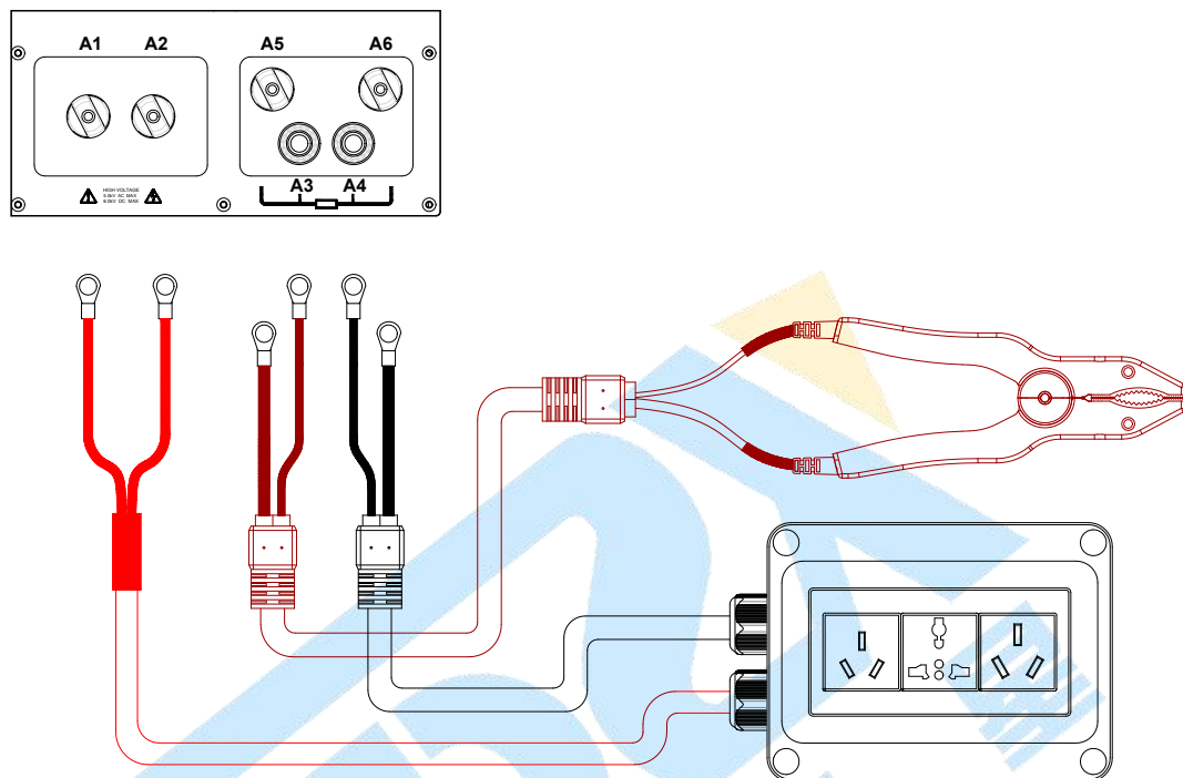
图 3-2-3-1 连接测试盒和接地测试钳
