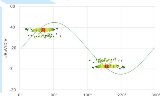
PRPD 图谱
