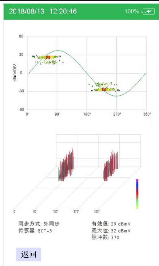
PRPD 与 PRPS 图谱
