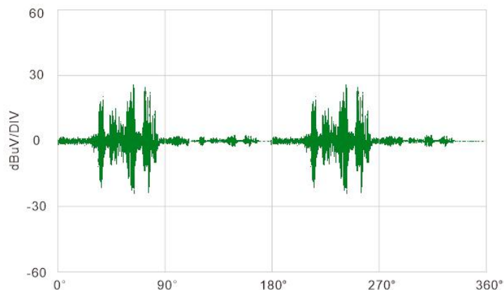
时域信号波形
