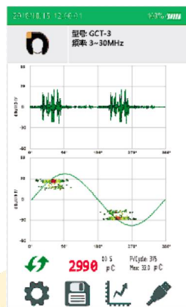
HFCT 测试界面
