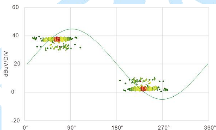
PRPD 图谱
